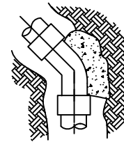
HORIZ. BEND
